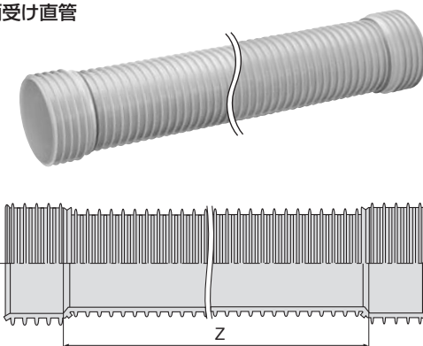
両受け直管
