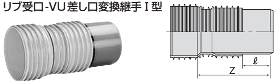
リブ受口-VU 差し口変換継手 I 型
